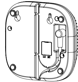
Raccordement électrique et emplacements de fixation sur le dessous
