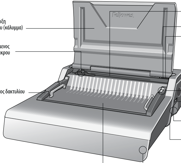
Αφαιρούμενη πλατφόρμα (κασέτα βιβλιοδεσίας)
