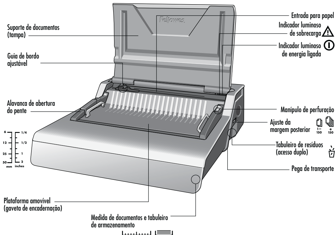
Armazenamento do pente e medida de documentos
